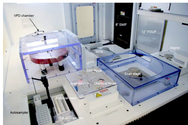
イアス社製品 Expert_PS モデルの内部 (シリコンウエハ表面上の金属元素を検査・分析・回収)
